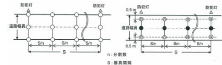
図2 生活道路等の水平面照度の測定位置 図3 生活道路等の鉛直面照度の測定位置
